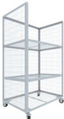
Cod: RLPROD695 CARRO UTILITARIO Tipo Jaula - 150x60x90cm - 3 Bandejas
